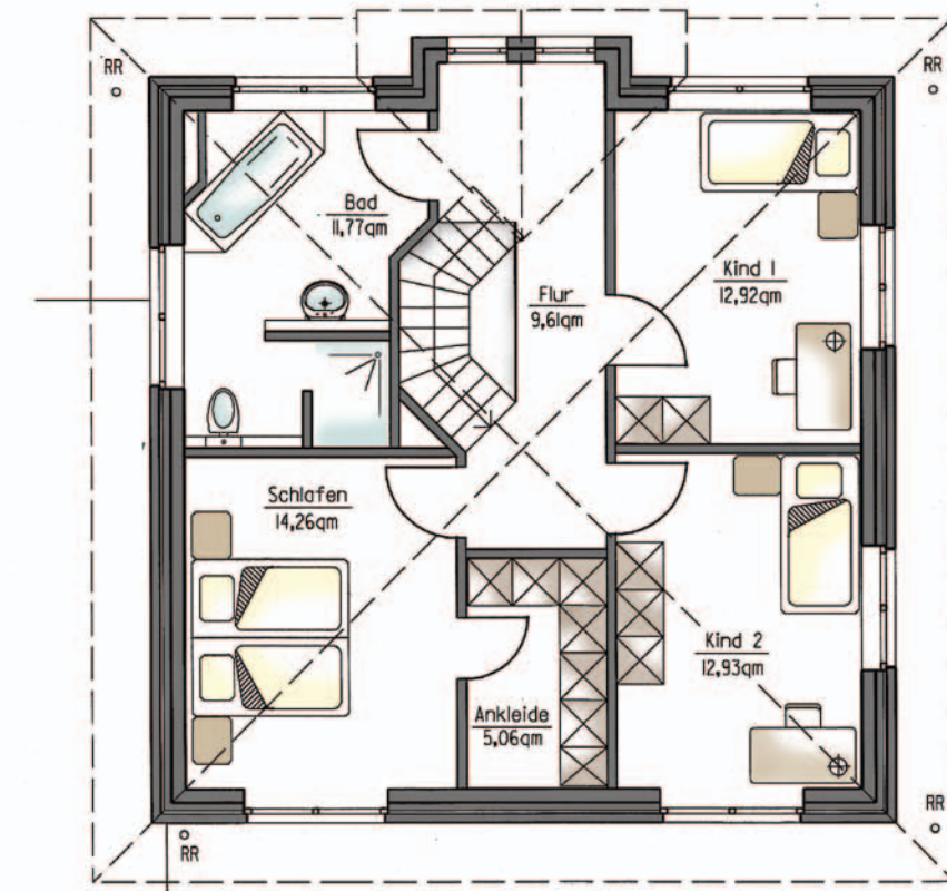
Grundriss Dachgeschoss
