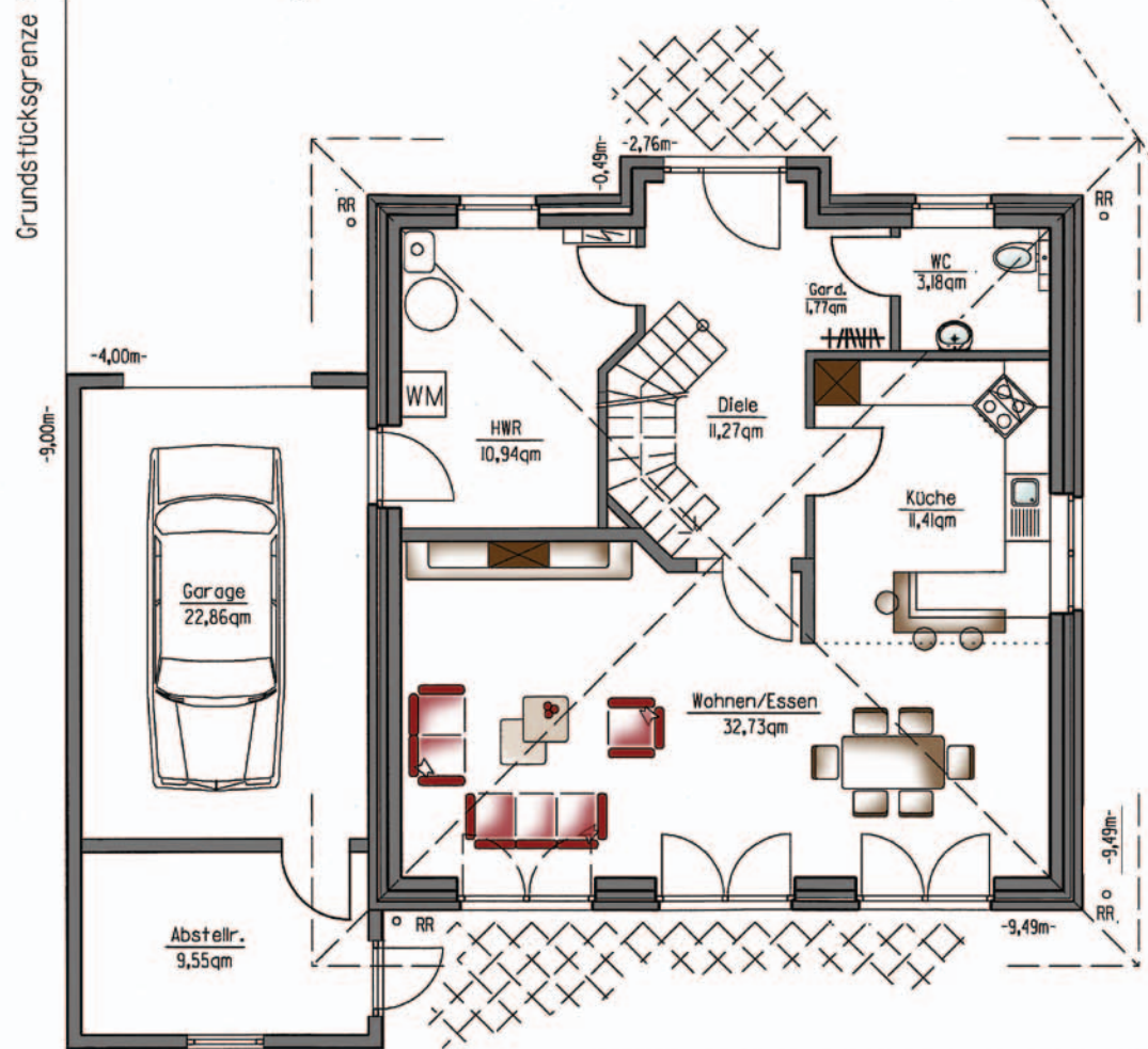
Grundriss Erdgeschoss
